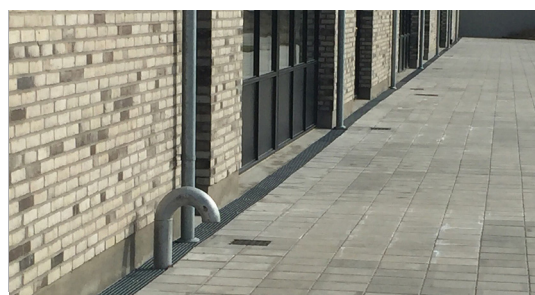
Med specialementet kan kloakudluftning eller nedløbsrør nemt passere sokkelrenden.
