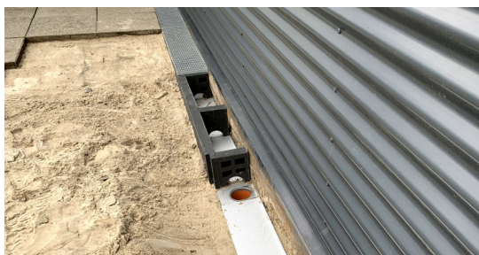
Bundplade og afløbselement lagt på afrettet underlag, derefter underdel og til sidst en rist.
