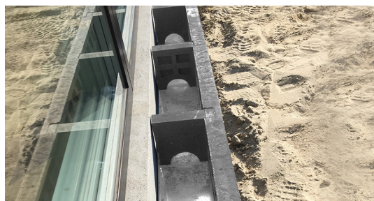
Underdelens buer sikrer at regnvandet frit løber til afløbselementet.
